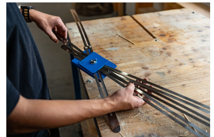
Grundplatte mit Winkelanschlag
