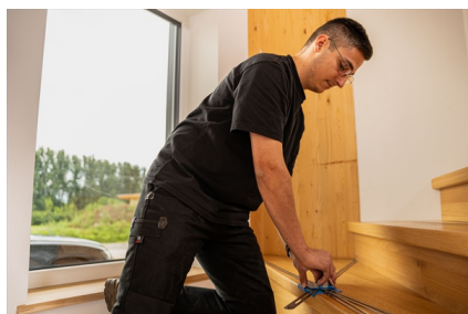
Scanner simple de la forme des marches.
