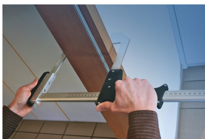
Medição exacta da espessura da parede ao agarrar à volta do mandril da porta
