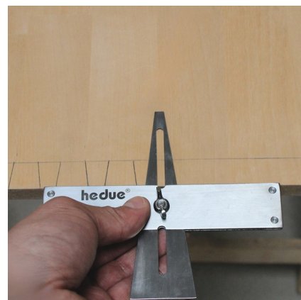
Fácil trazado de ensambles cola de milano y cola de milano
