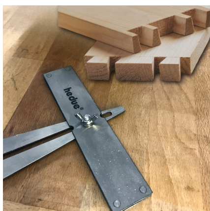
La lengua tiene una inclinación de 1:8
