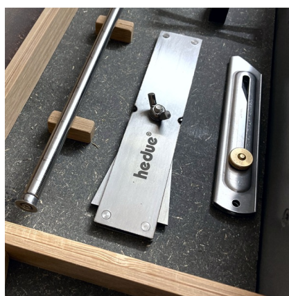
Możliwość obrotu o 90° ułatwia przechowywanie.
