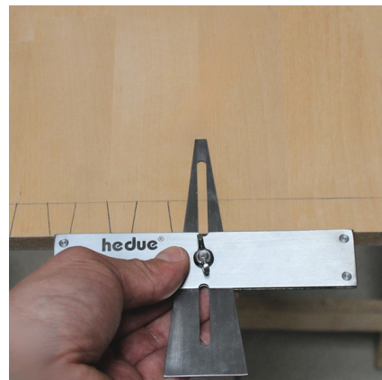
Trasare ușoară a îmbinărilor în dinți și în coadă de rândunică
