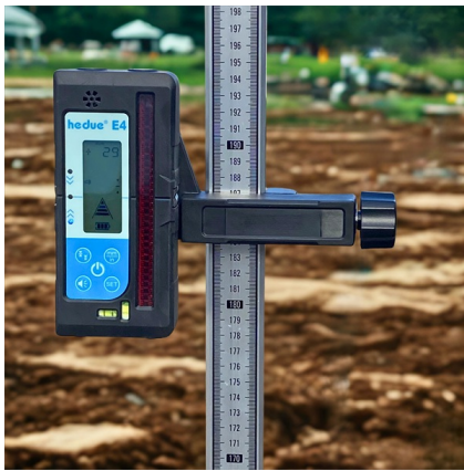
Cyfrowy odbiornik laserowy pokazuje różnicę wysokości względem linii laserowej w mm lub calach.
