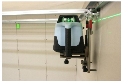
Meilleure visualisation de la ligne laser à l'intérieur grâce à la diode laser verte.
