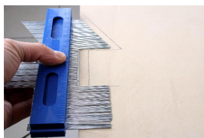
La línea de perfil escaneada puede transferirse fácilmente a una pieza de trabajo gracias al soporte plano
