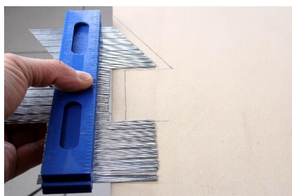
Linia de profil eșantionată este de reprodus pe o piesă de lucru, datorită reazemului plat și neted
