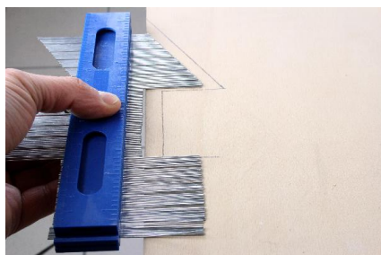
Die abgetastete Profillinie ist dank der flachen Auflage leicht auf ein Werkstück übertragbar
