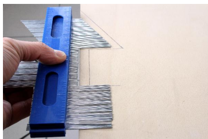
De gescande profiellijn kan eenvoudig op een werkstuk worden overgebracht dankzij de vlakke ondersteuning
