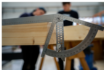
O Ângulo alfa pode ser utilizado para todos os tipos de carpintaria.
