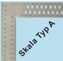
Zimmermannswinkel hedue ZV 800 mm mit mm-Skala Typ A und Anreißlöcher, Art.-Nr. V082
