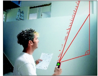
Indirekt távolságmérés
