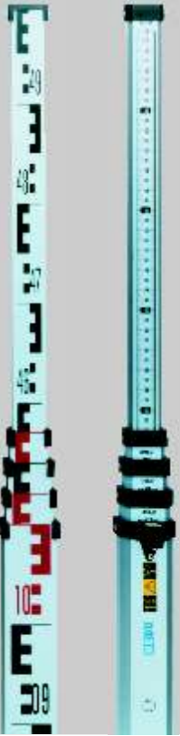
Avec niveau à boîte et etui.
